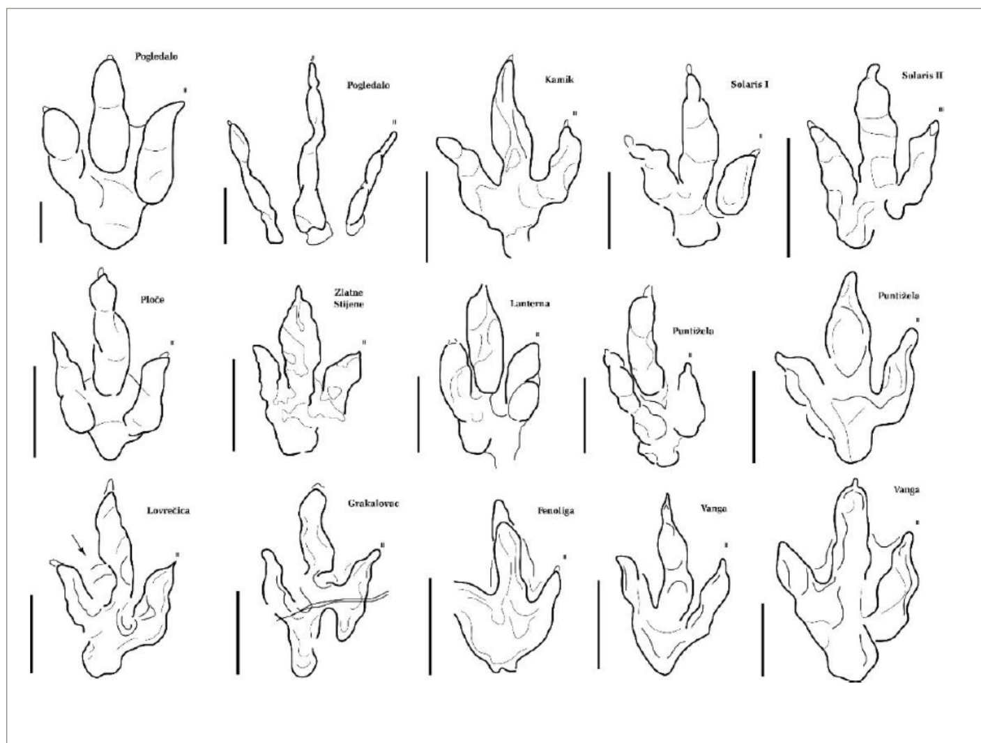
Slika 22: Otisci stopala teropoda s nalazišta na AdCP-u; mjerilo = 10 cm.
