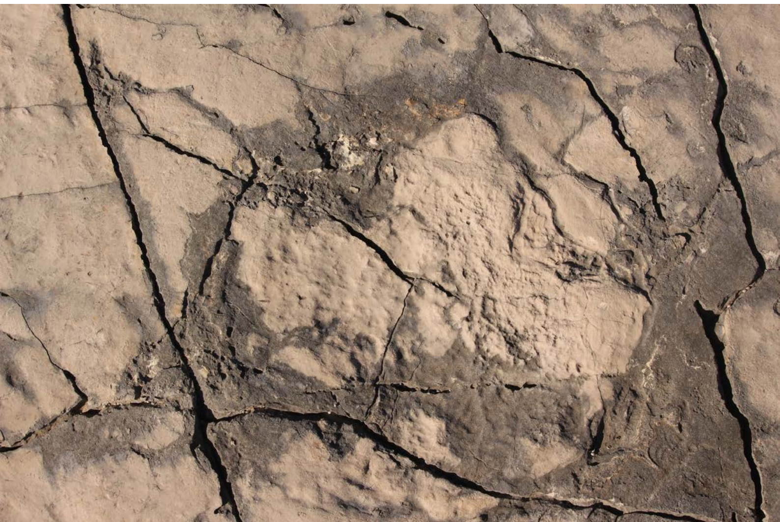
Slika 26: Fosilni trag stopala ornitopodnog dinosaura s nalazišta Kamik/Plješivac, gornji alb, starija kreda, starosti 105 milijuna godina, Veli Brijun; autor fotografije: Damir Pocrnić
