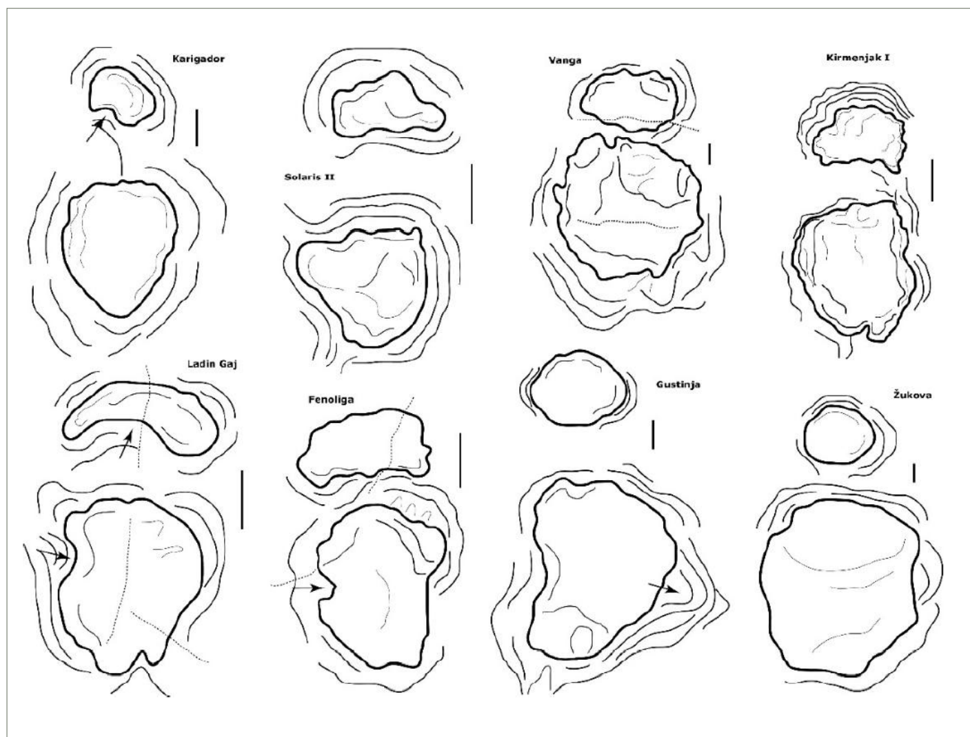
Slika 21: Otisci stopala sauropoda s nalazišta na AdCP-u; mjerilo = 10 cm.
